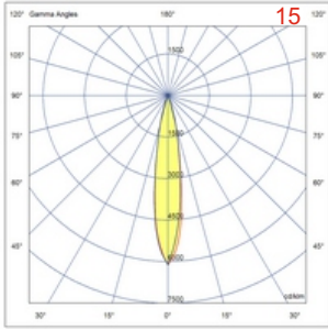
Lens Işık Yayılm Açıları
